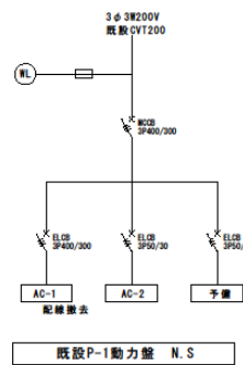
既設P-1動力盤 N.S
