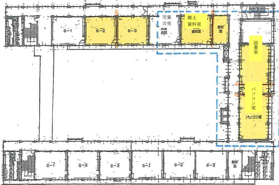
3階平面図
