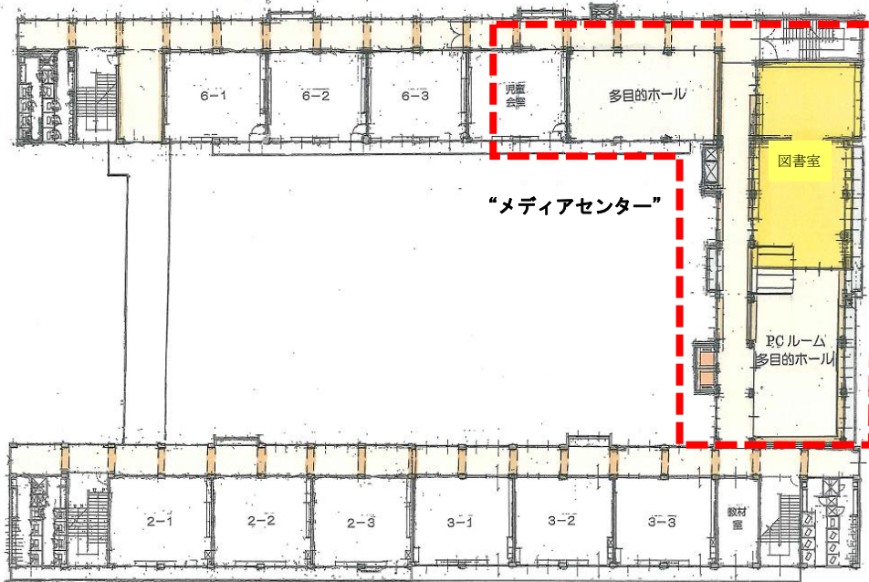
3階平面図
