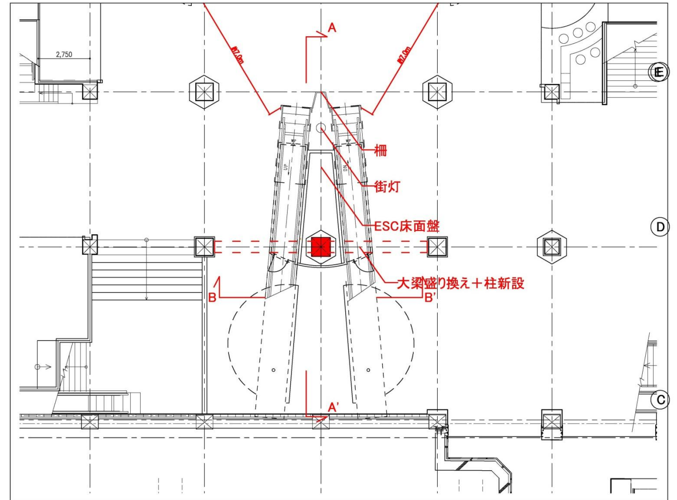
地下1階平面図
