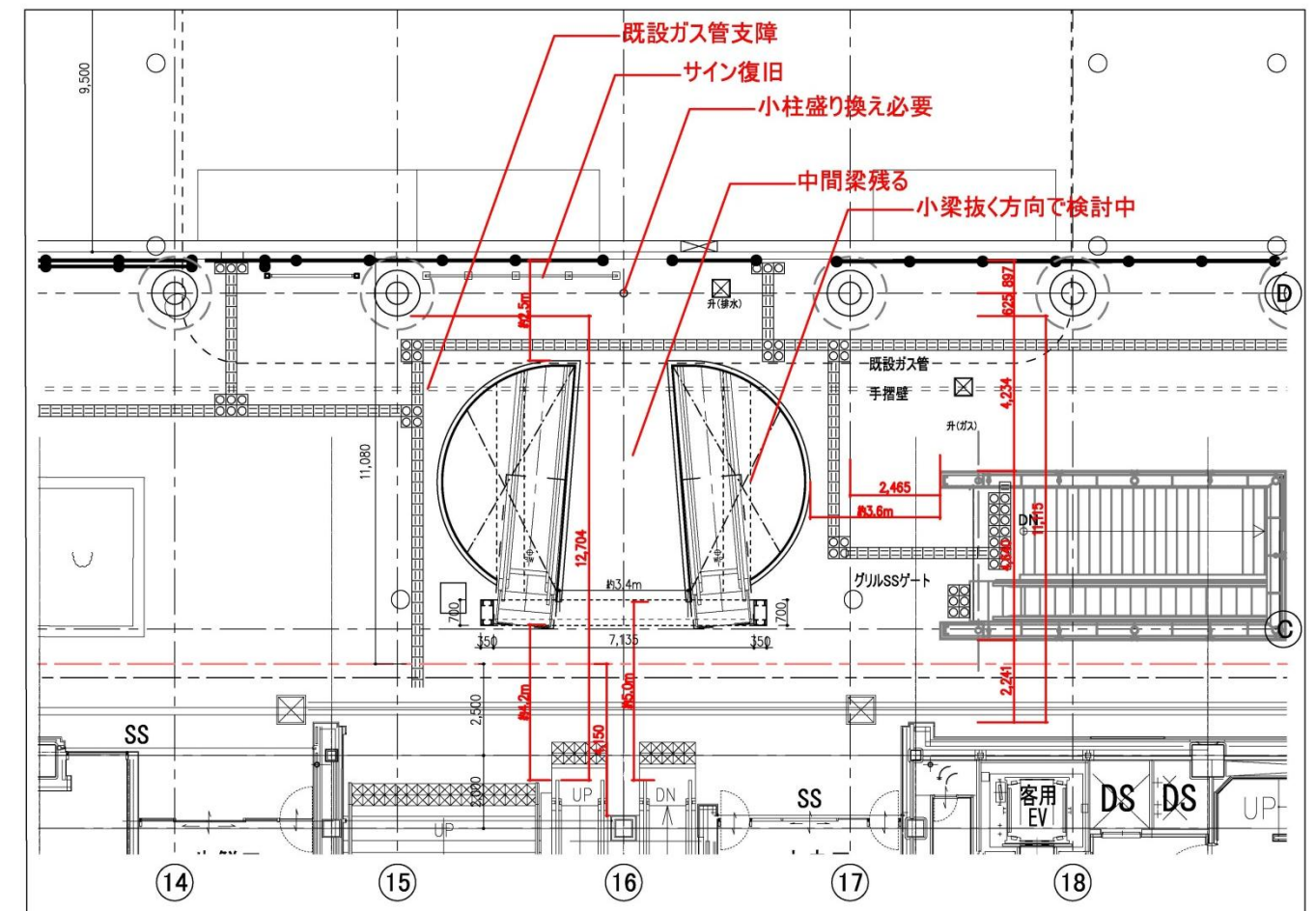
1階平面図
