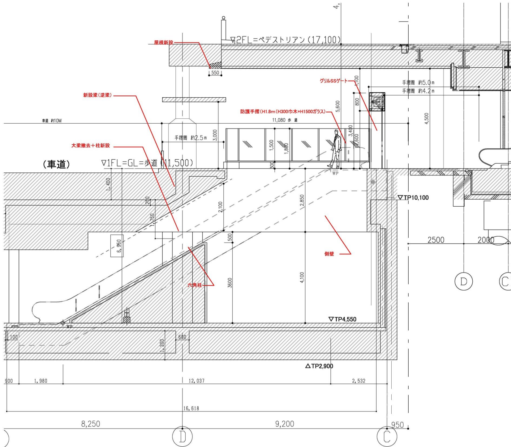
A-A' 断面図
