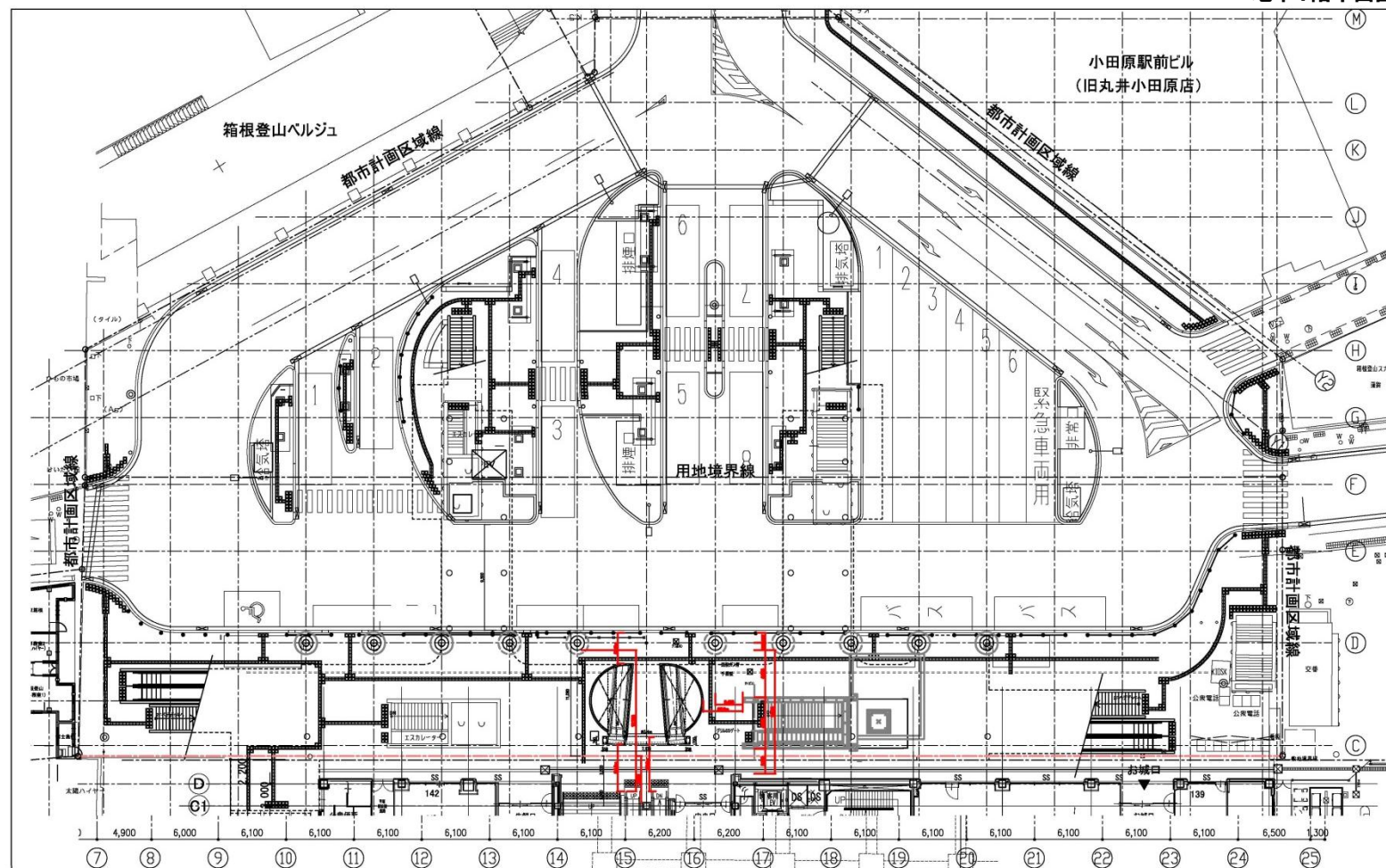
1階平面図
