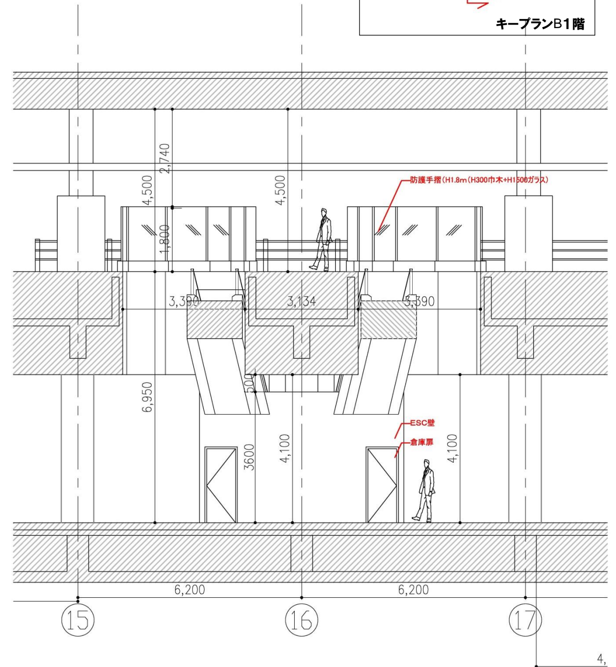
B-B' 断面図
