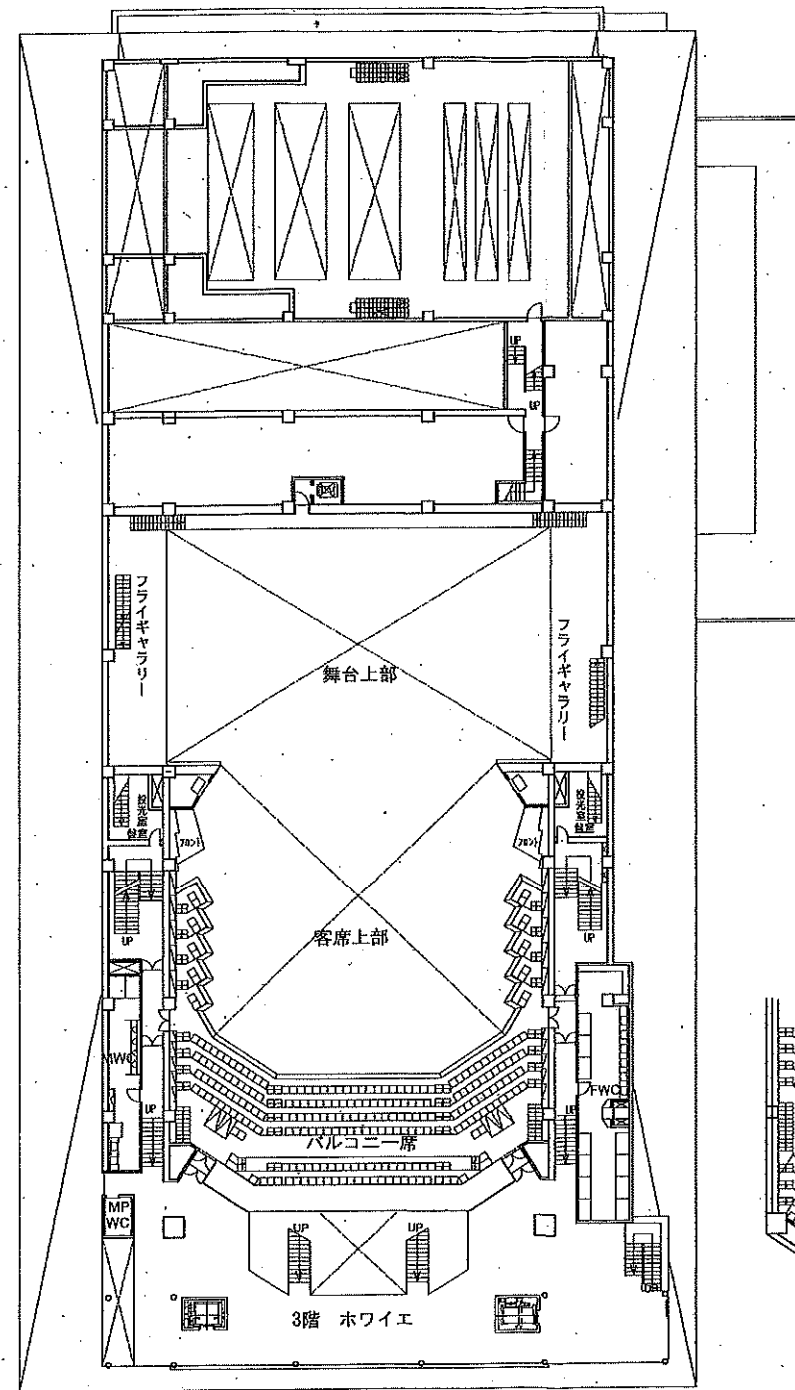
3F 平面図 1:500
