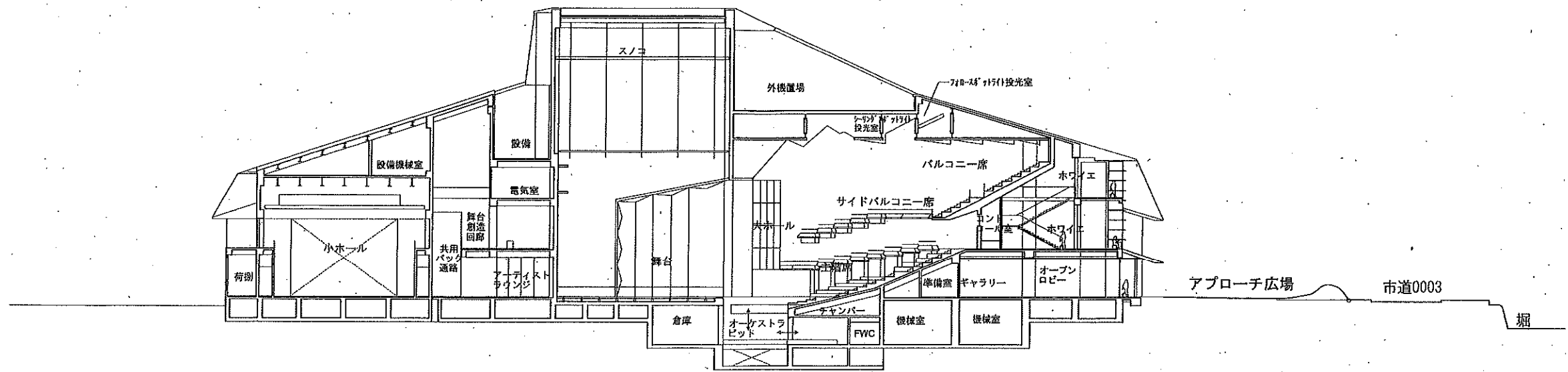
断面図 1:500
