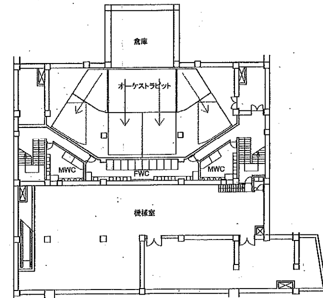
B1F 平面図 1:500
