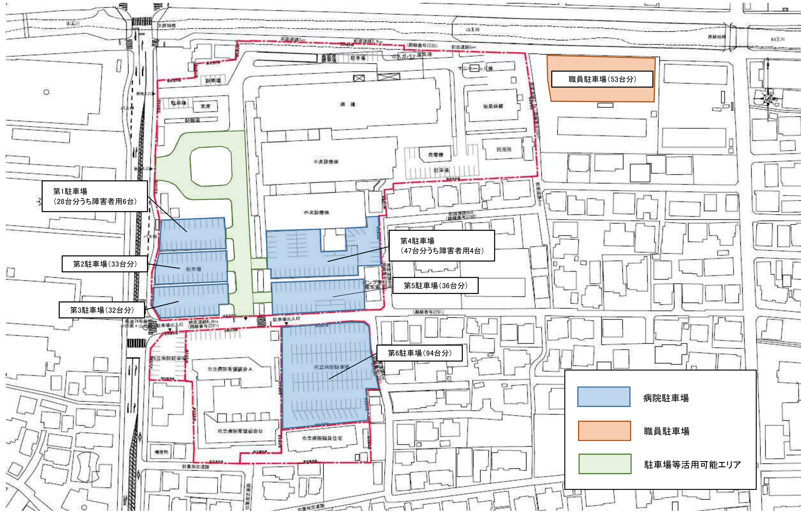
配置図
