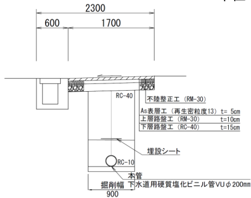
標準横断面
