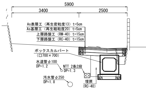
標準横断面
