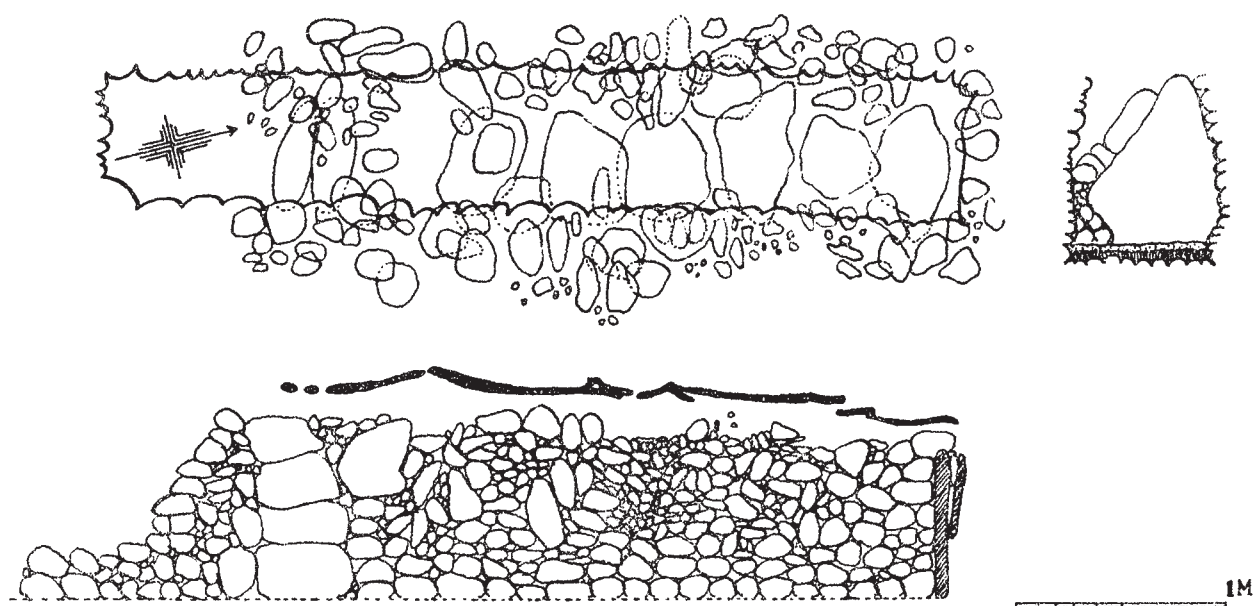
第8図 久野4号墳石室実測図（1/50）
