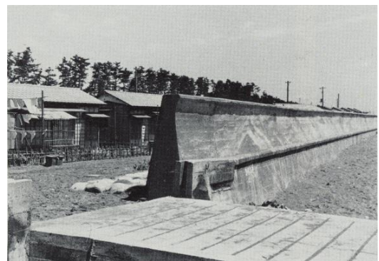
1-44 西湘バイパス整備前の海岸堤防
