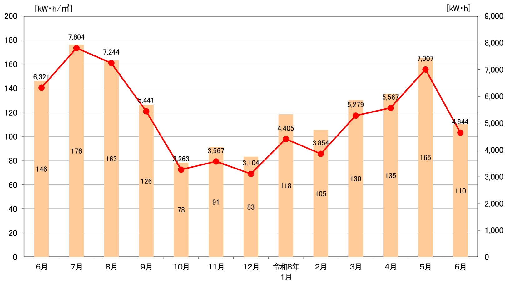
図. 市役所にある太陽光発電システム(60kW)の発電量と日射量との関係 (令和7年6月～令和8年6月)
