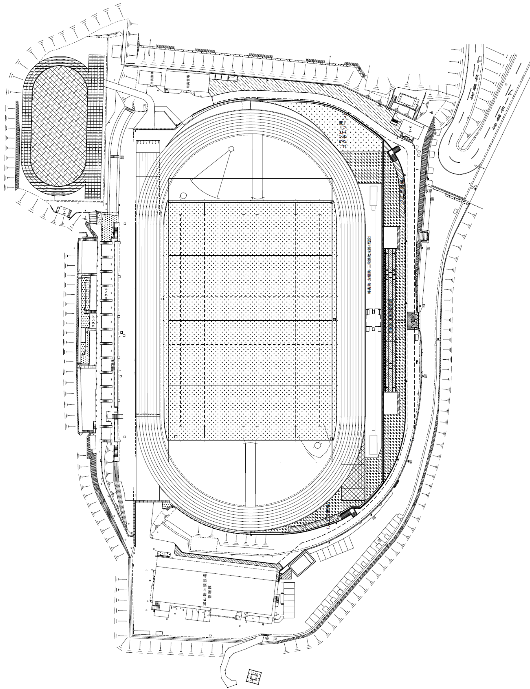
城山陸上競技場 平面図
