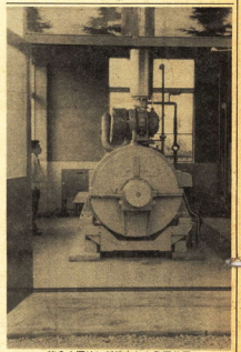
第二水源地に新設された発電装置
