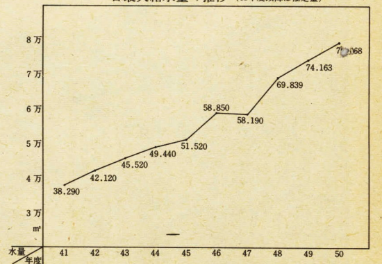
一日最大給水量の推移 (48年度以降は推定量)
