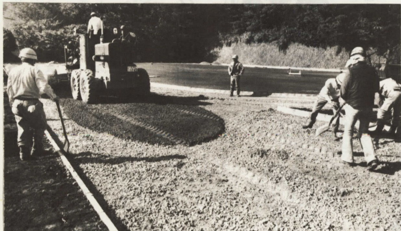
アスファルト舗装の上にウレタンの弾性床が張られ、雨天時も使用が可能になる
