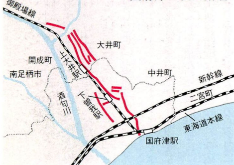
国府津・松田断層
