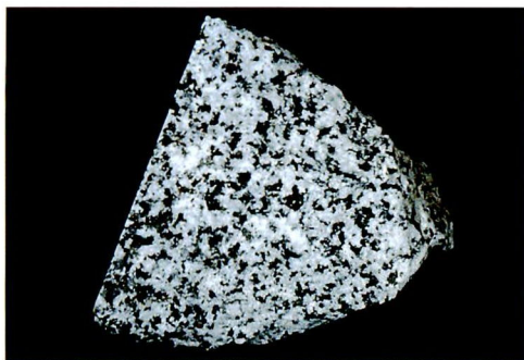
丹沢山地の中心部に露出する石英閃緑岩。トータル岩とも呼ばれる。
