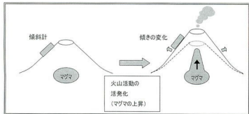
マグマの上昇による山体の隆起・膨張のイメージ
