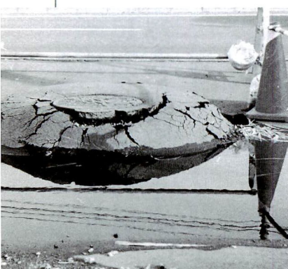
平成15年十勝沖地震での液状化現象による被害例
