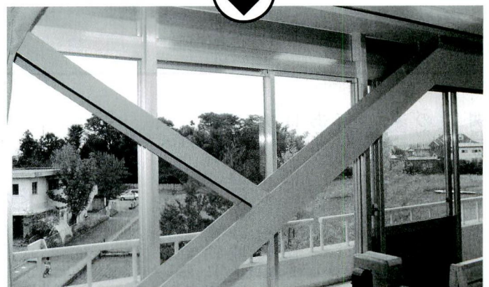
耐震補強工事で鉄柱が取り付けられた窓。外の景色は見づらくなったが、地震には格段に強くなった。
