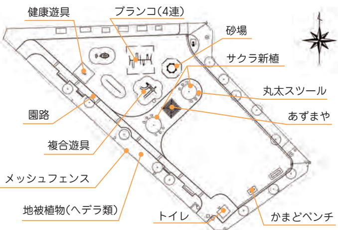
南鴨宮駅前公園の再整備計画図
