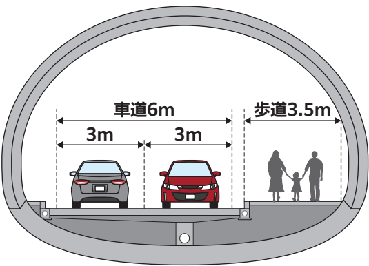
▲新坂下トンネルの横断面図
