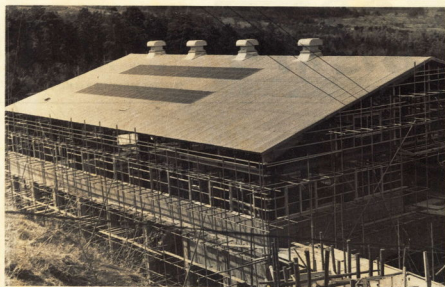
じんかい焼却場 市内府川(諏訪原コンポスト隣地)に昭和40年度から2カ年の工期で着工。 本年秋ごろに完成の予定。総工費1億1,787万円、処理能力1日に65トン。
