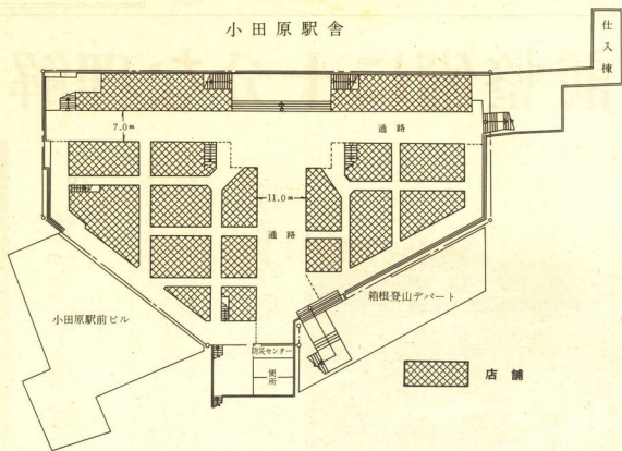
小田原駅東口広場地下街完成予想図(広場から地下1階を透視)
