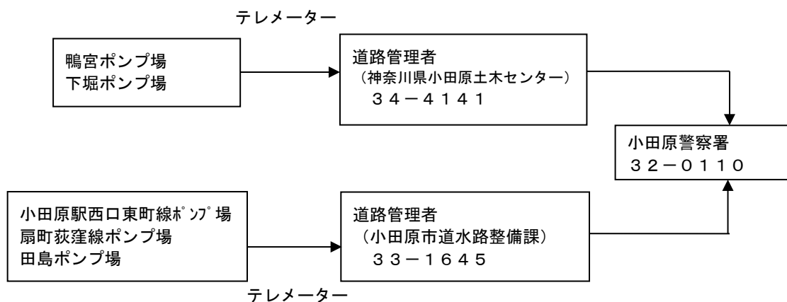
連絡系統図
