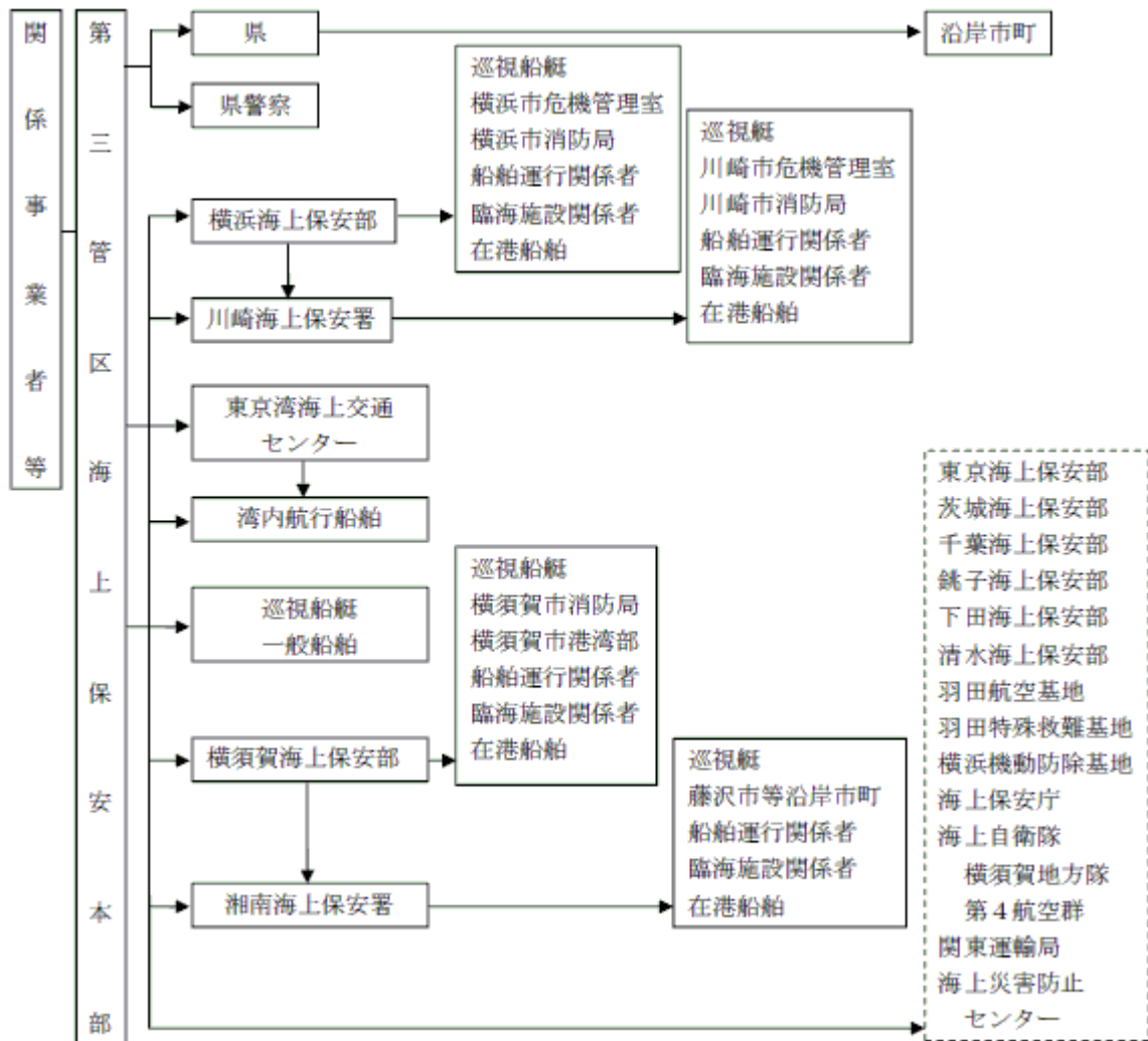
資料 14-3 船舶等の事故発生時の連絡系統図
