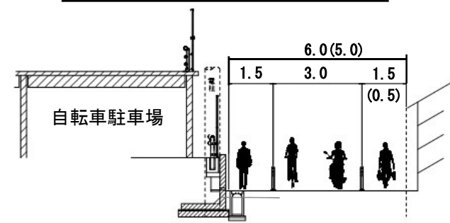
横断図1 (市道4294)
