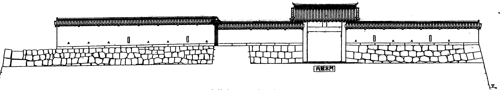
全体立面図・内冠木門
