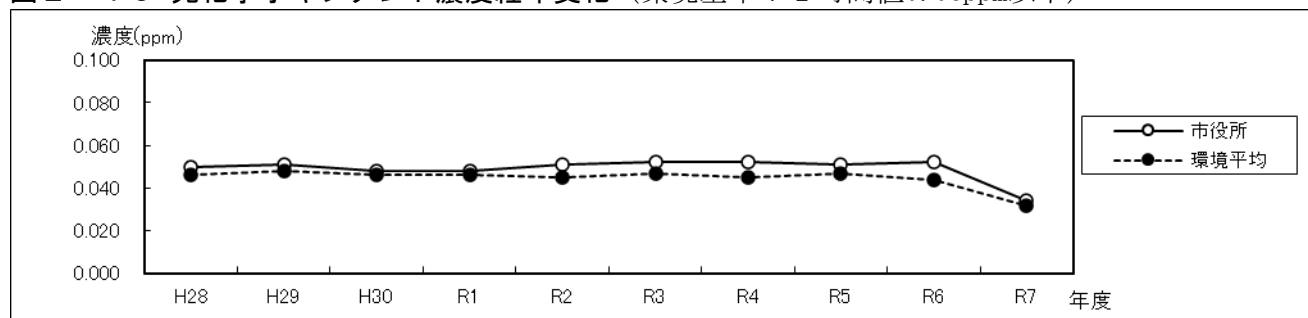
図Ⅱ－10 光化学オキシダント濃度経年変化（環境基準：1時間値0.06ppm以下）
