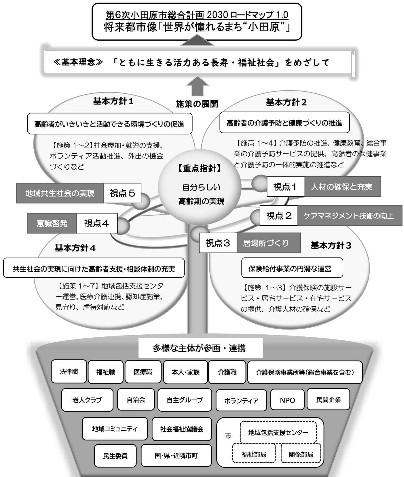
図3-2 施策の体系
