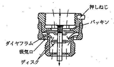
(3) ホース接続形(カップリング水栓用)
