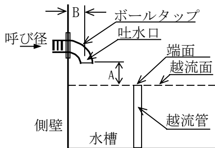
図 4-6-6 越流管（縦取出）
