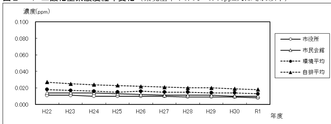
図Ⅱ-4 二酸化窒素濃度経年変化 (環境基準: 0.04~0.06ppm又はそれ以下)
