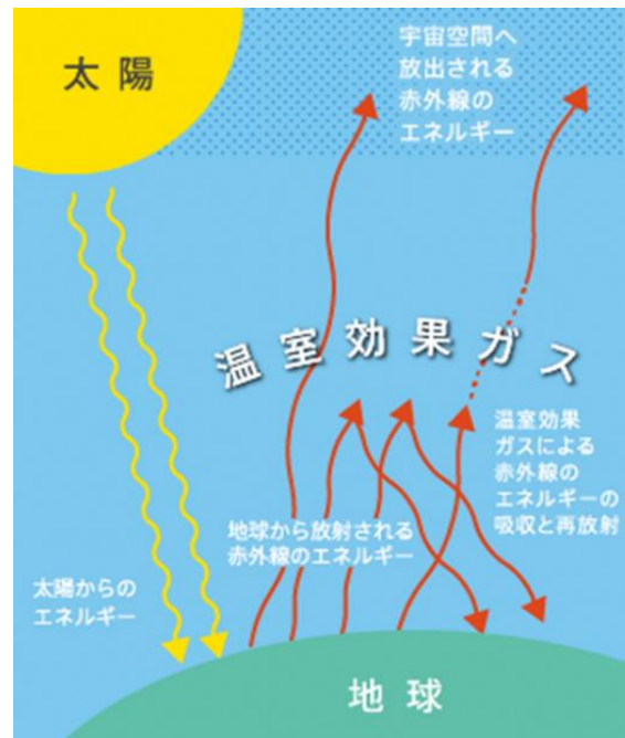
『地球温暖化のメカニズム』 出典：環境省ホームページ
