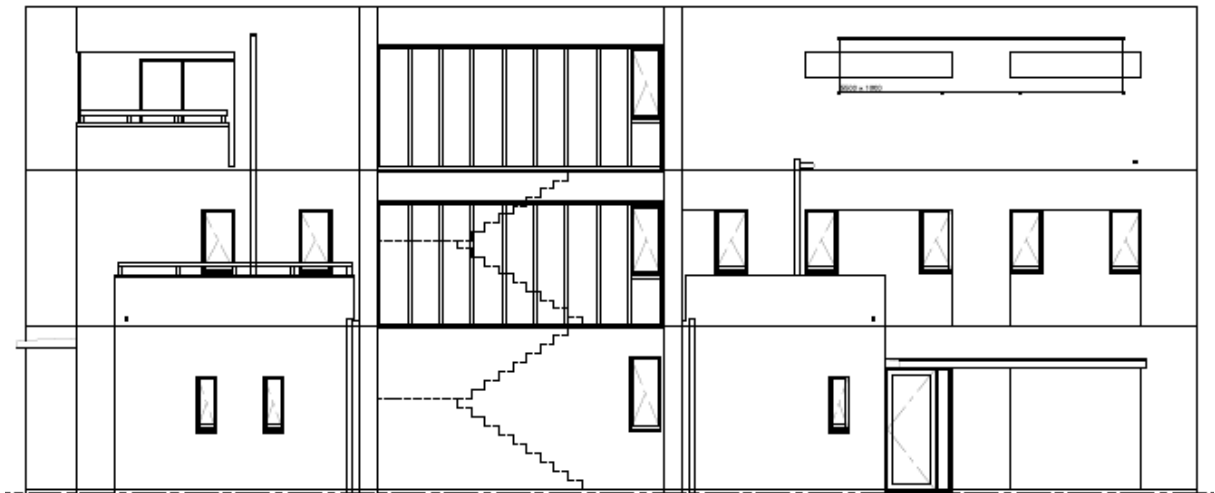
北立面图
