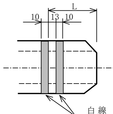
図 4-6-4 差し口白線位置図
