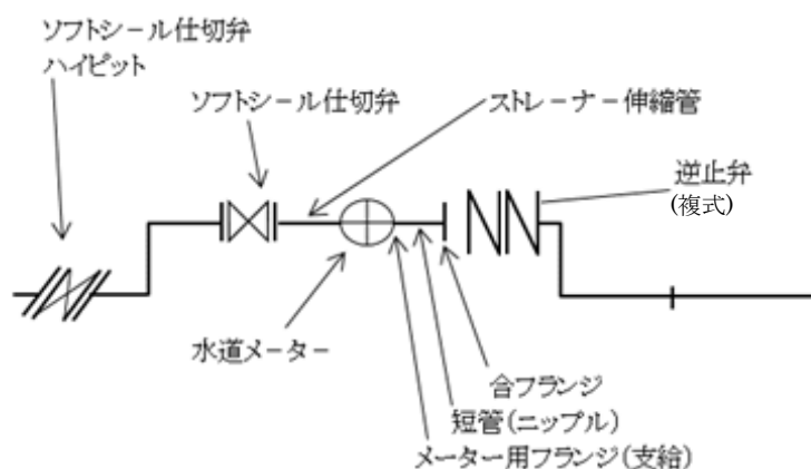
水道メーター口径 \phi 50 \sim
