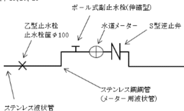
水道メーター口径 \phi 13, 20, 25
