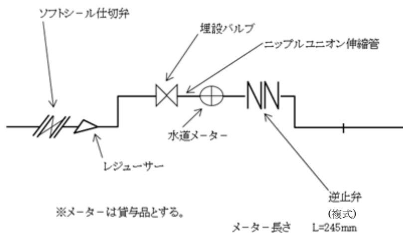
水道メーター口径 \phi 40
