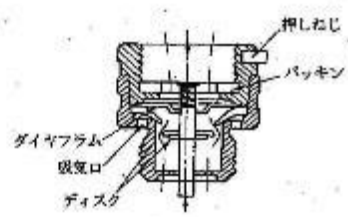
(3) ホース巻戻形 (カップリング水栓用)
