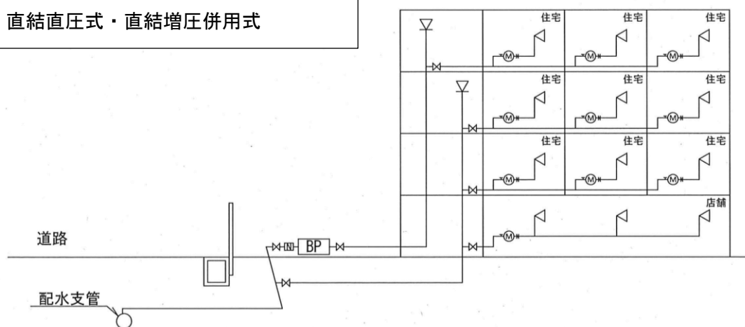
図 2-4-3 直結式の例
