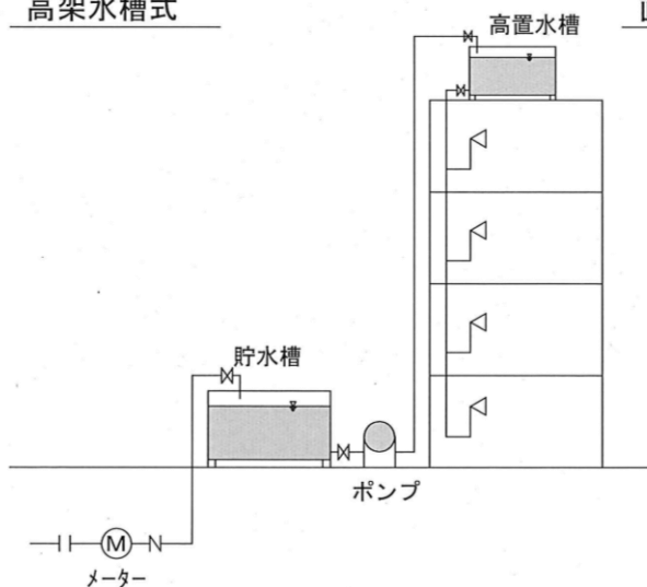
高架水槽式
