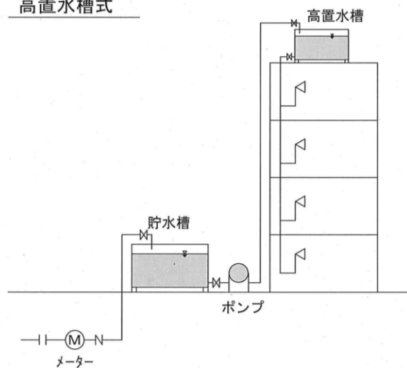
高置水槽式
