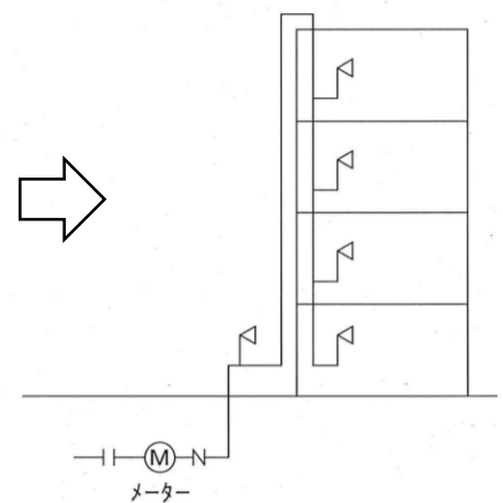
直圧式
