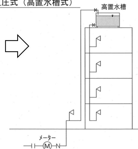
直圧式 (高置水槽式)
