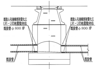
じしんたいさくこうじ 地震対策工事イメージ図
