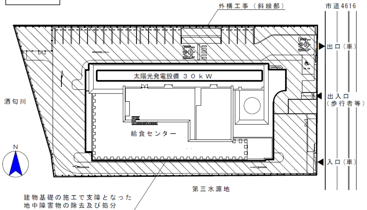
配置図
