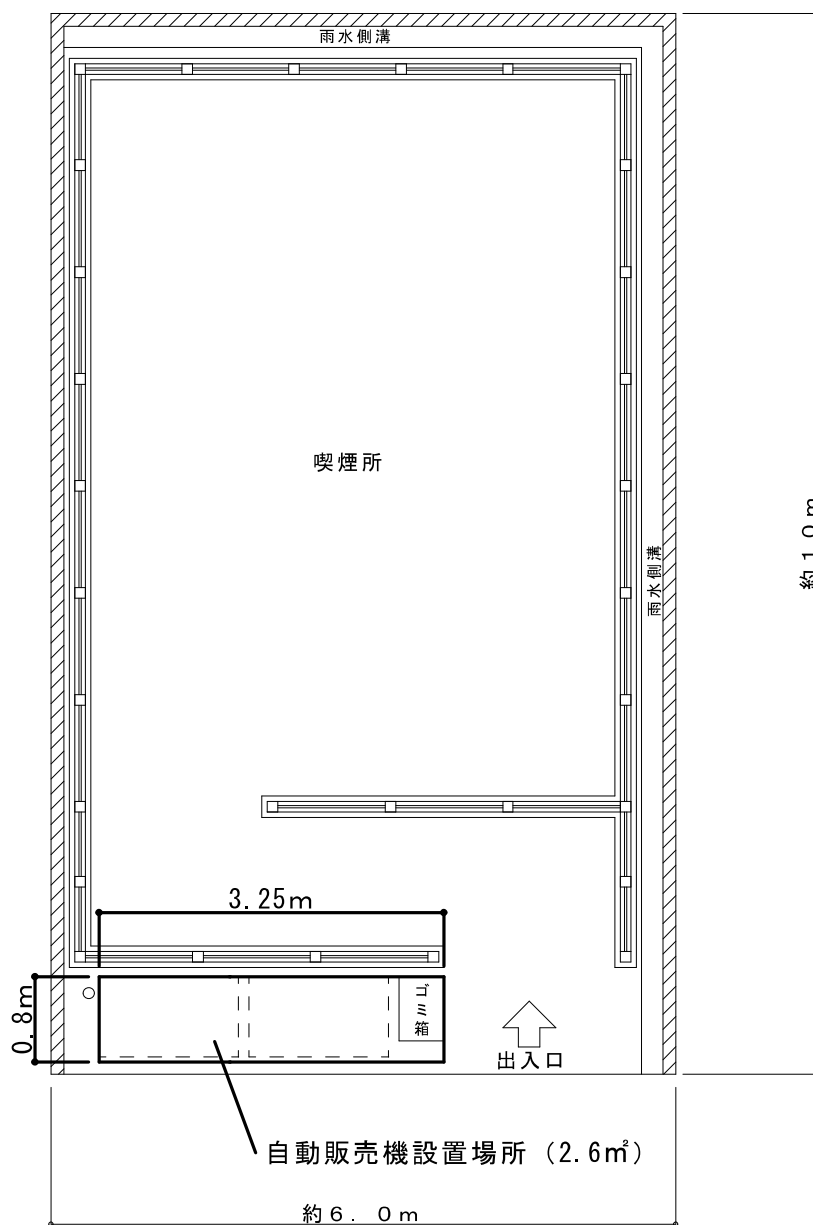
平面図
