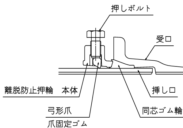
図 2-18 K 形特殊押輪(3DkN 以上)継手構造
