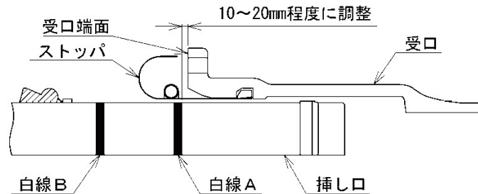
図 2-14 挿し口の挿入
