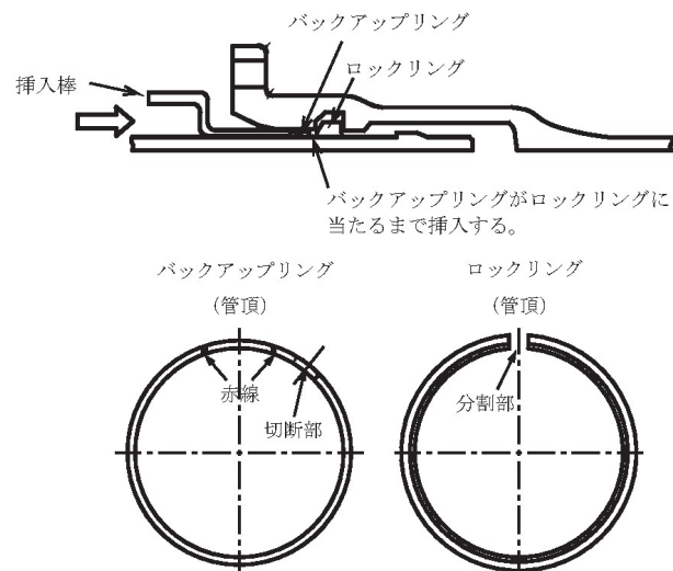
図 2-15 バックアップリングの挿入
