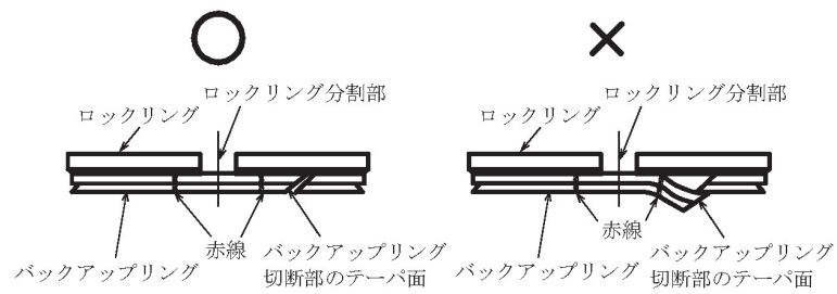
図 2-16 バックアップリング切断部の確認
