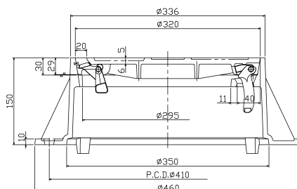
仕切弁室工（ハイピット（参考 D_p=1100 ））
