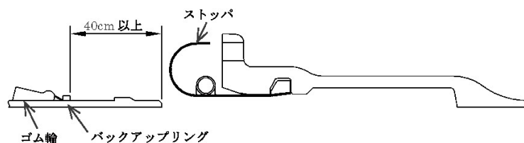
図 2-13 接合部品のセット位置
