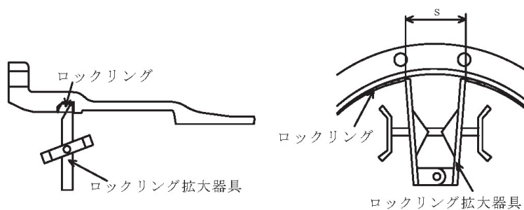
図 2-10 ロックリング拡大器の装着
