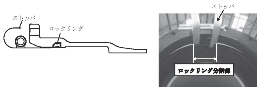
図 2-12 ストッパーの装着
