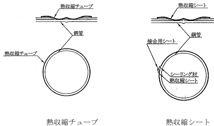
図 2-19 ジョイントコート
