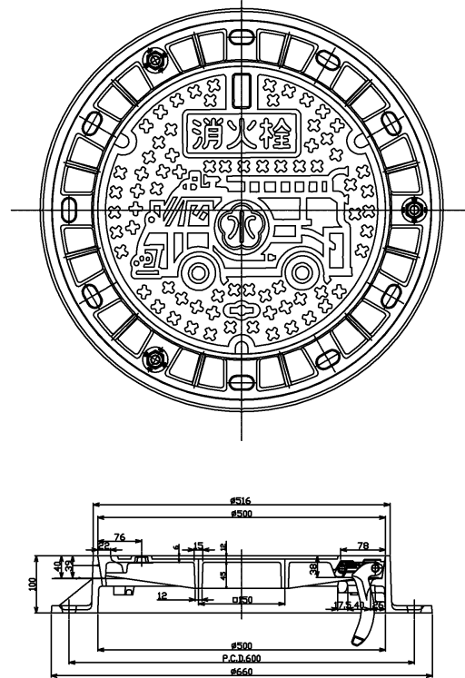
消火栓表筐
