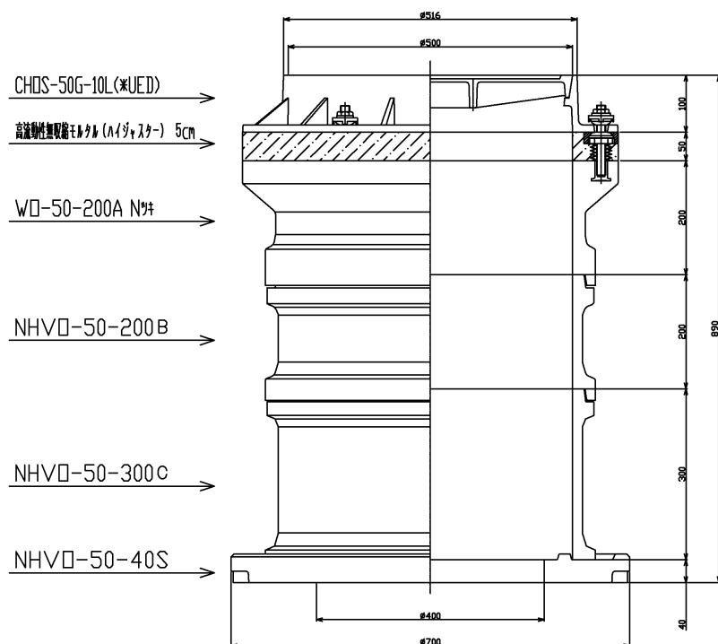
空気弁室工（ハイジヤスター）
