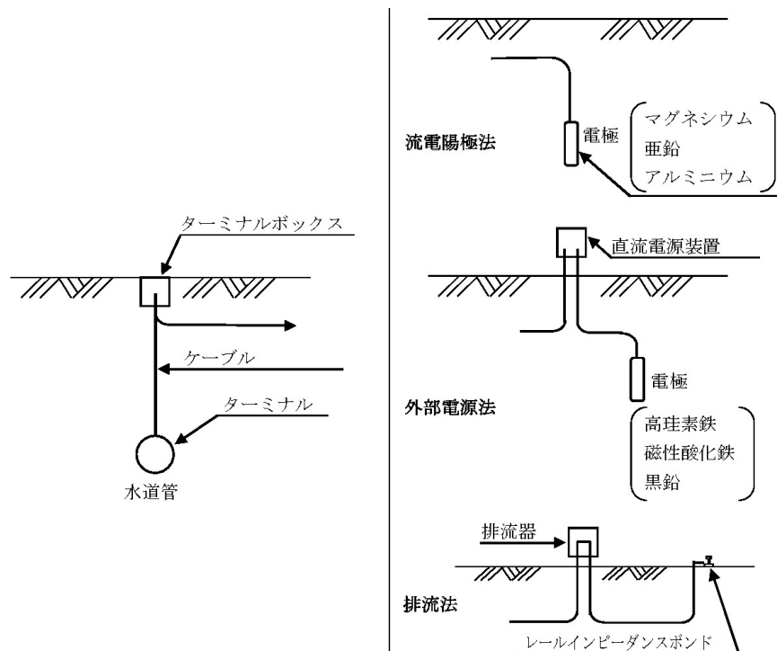
図 2-20 防食装置参考図
