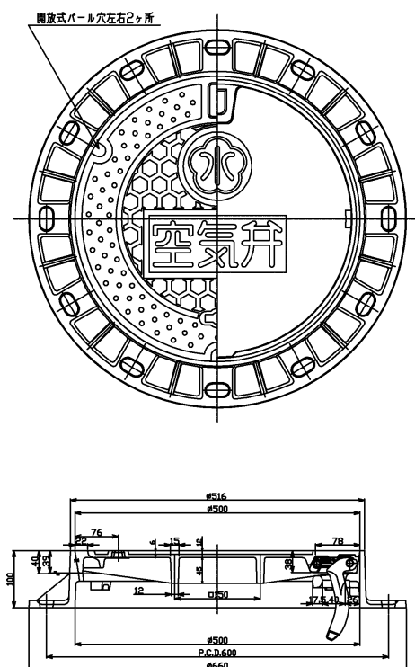
空気弁表筐
