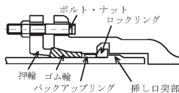
図 2-9 NS 形継手構造
