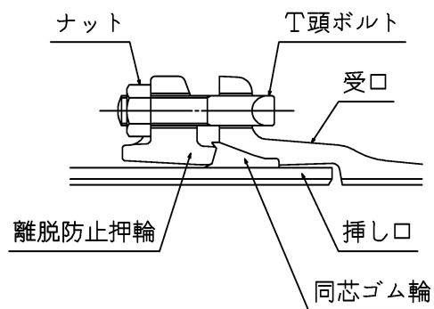
図 2-17 K 形継手構造
