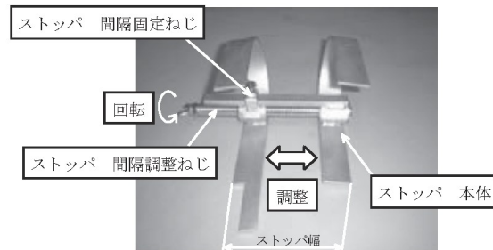
図 2-11 ストッパーの概要
