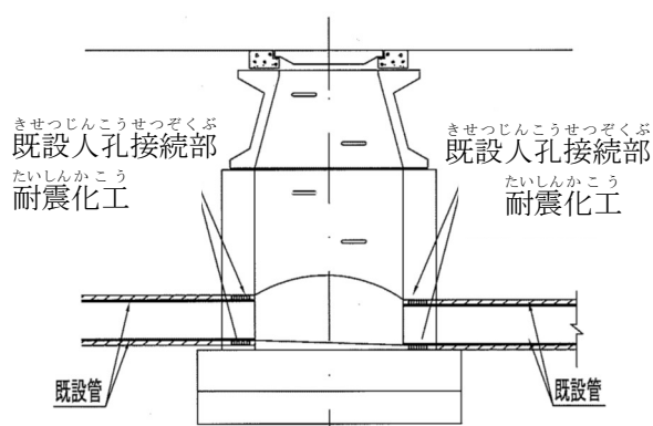
じしんたいさくこうじ ず 地震対策工事イメージ図
