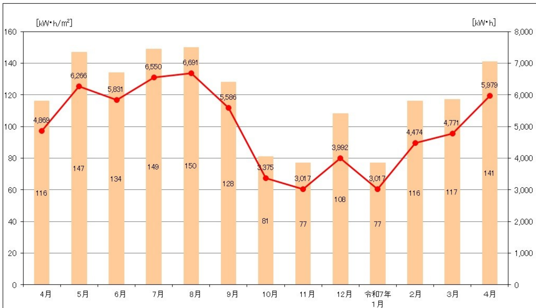
図. 市役所にある太陽光発電システム(60kW)の発電量と日射量との関係 (令和6年4月～令和7年4月)
