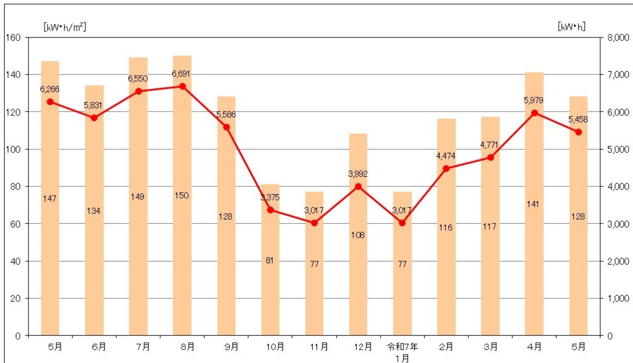
図. 市役所にある太陽光発電システム(60kW)の発電量と日射量との関係 (令和6年5月～令和7年5月)
