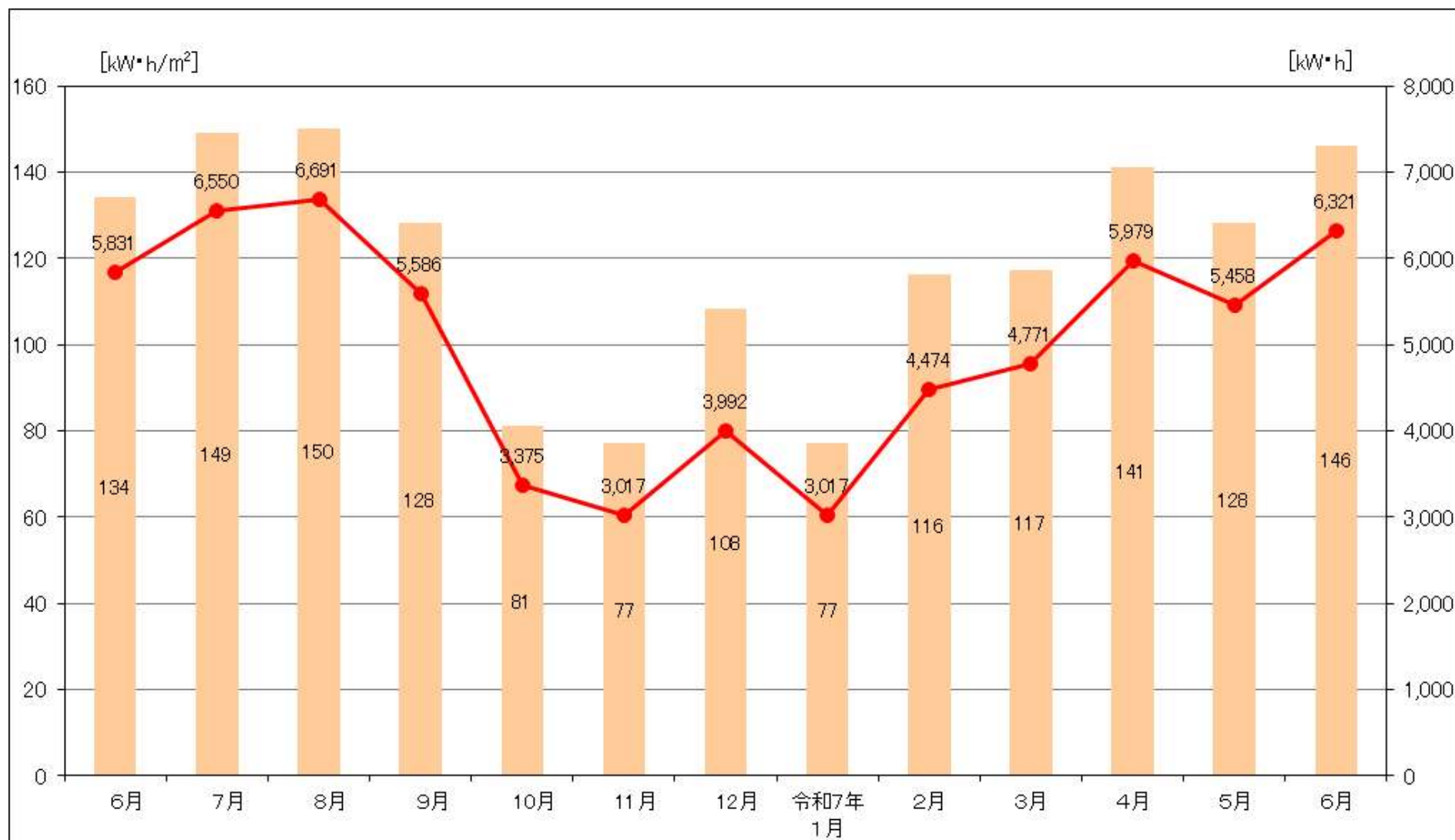
図. 市役所にある太陽光発電システム(60kW)の発電量と日射量との関係 (令和6年6月～令和7年6月)
