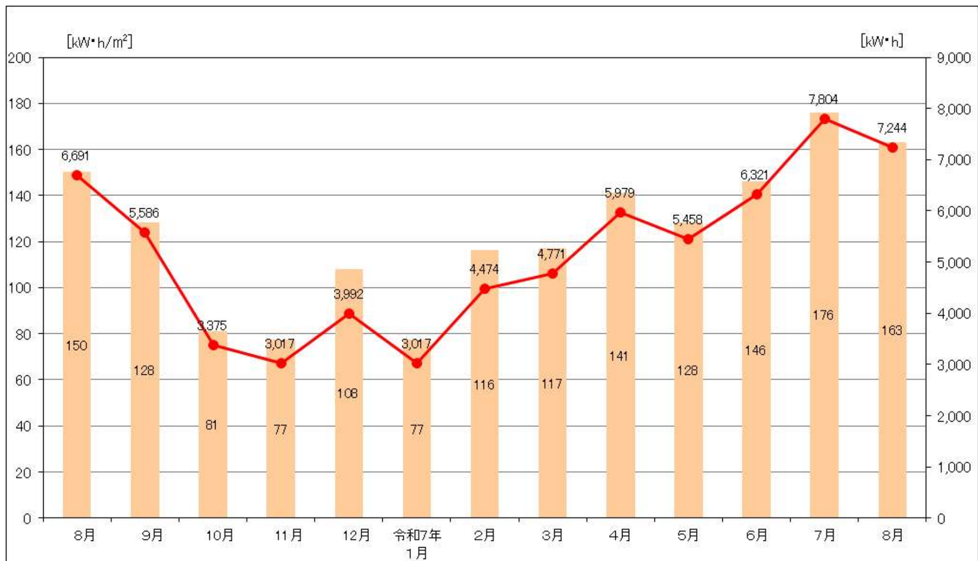
図. 市役所にある太陽光発電システム(60kW)の発電量と日射量との関係 (令和6年8月～令和7年8月)
