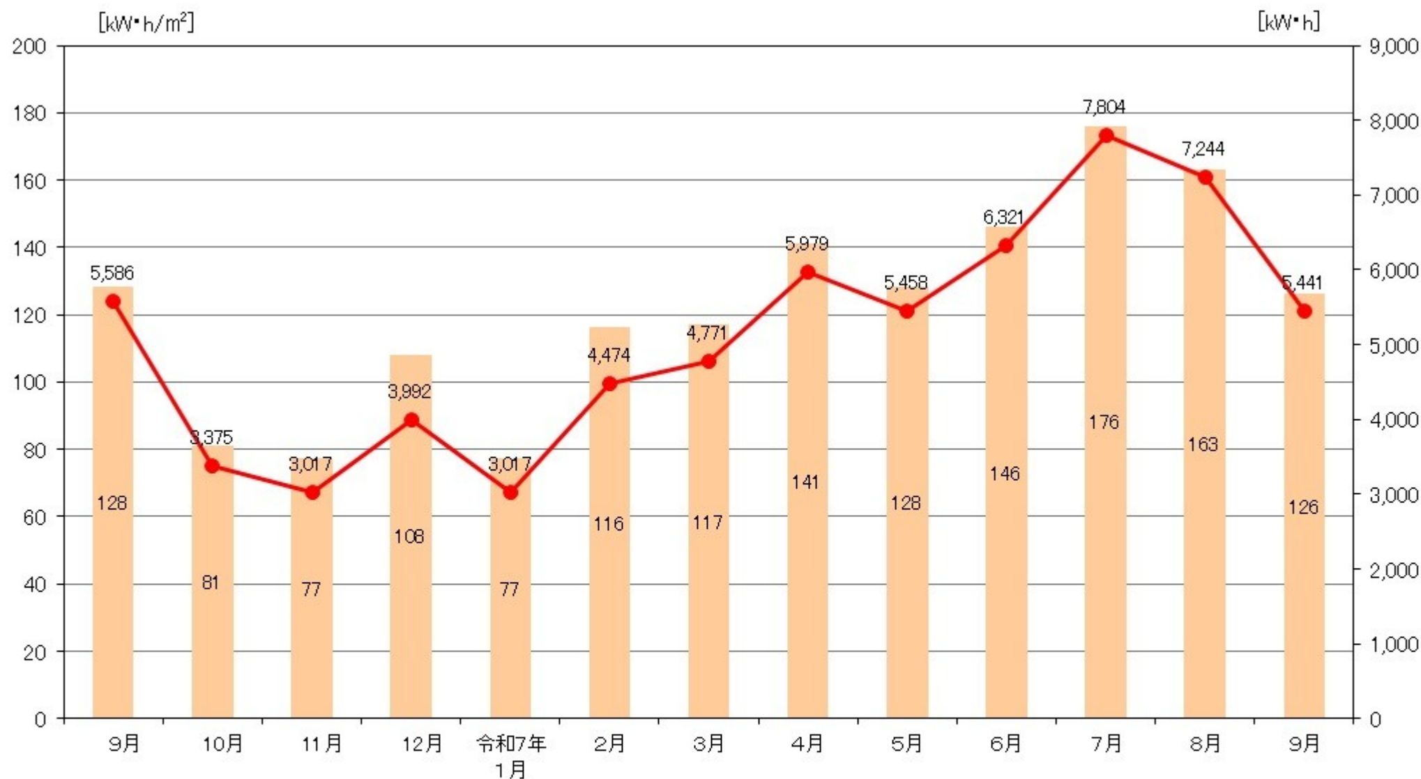
図. 市役所にある太陽光発電システム(60kW)の発電量と日射量との関係 (令和6年9月～令和7年9月)
