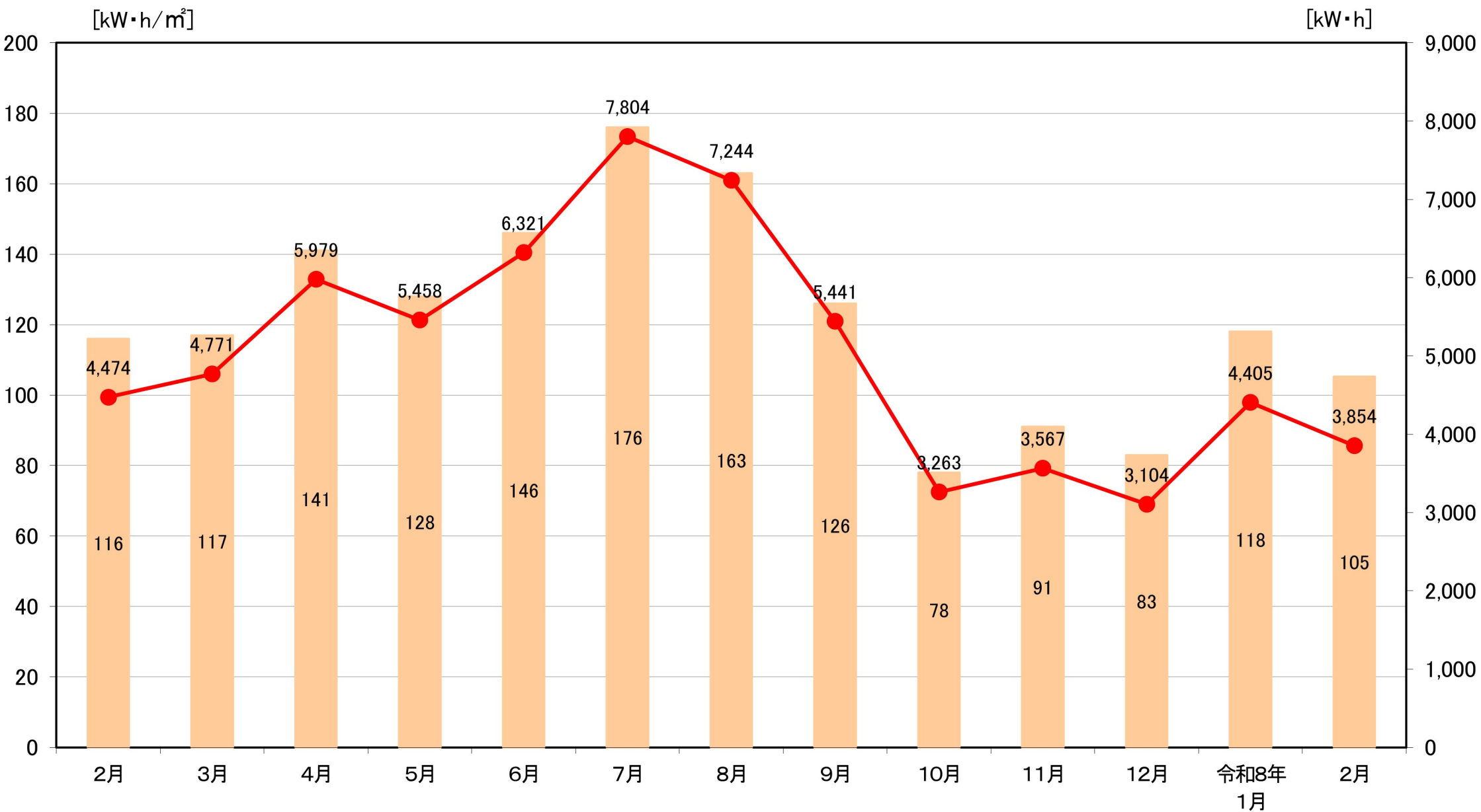
図. 市役所にある太陽光発電システム(60kW)の発電量と日射量との関係 (令和7年2月～令和8年2月)
