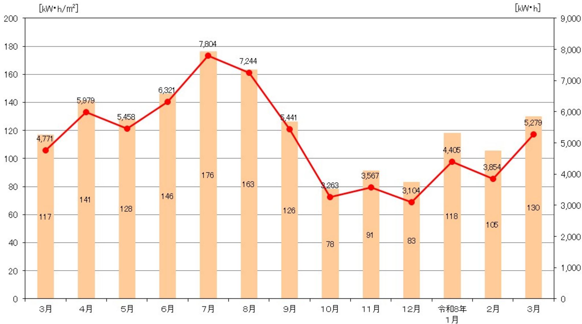
図. 市役所にある太陽光発電システム(60kW)の発電量と日射量との関係 (令和7年3月～令和8年3月)
