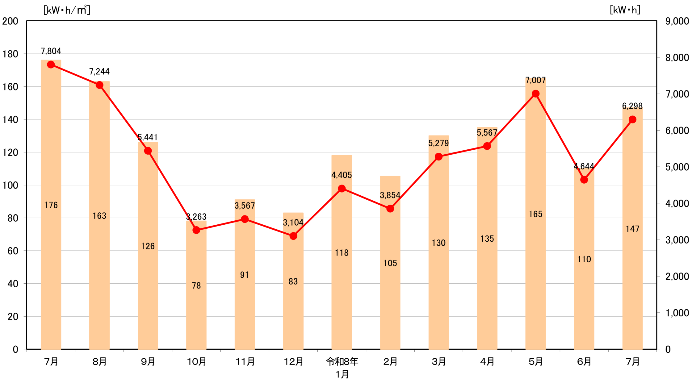
図. 市役所にある太陽光発電システム(60kW)の発電量と日射量との関係 (令和7年7月～令和8年7月)
