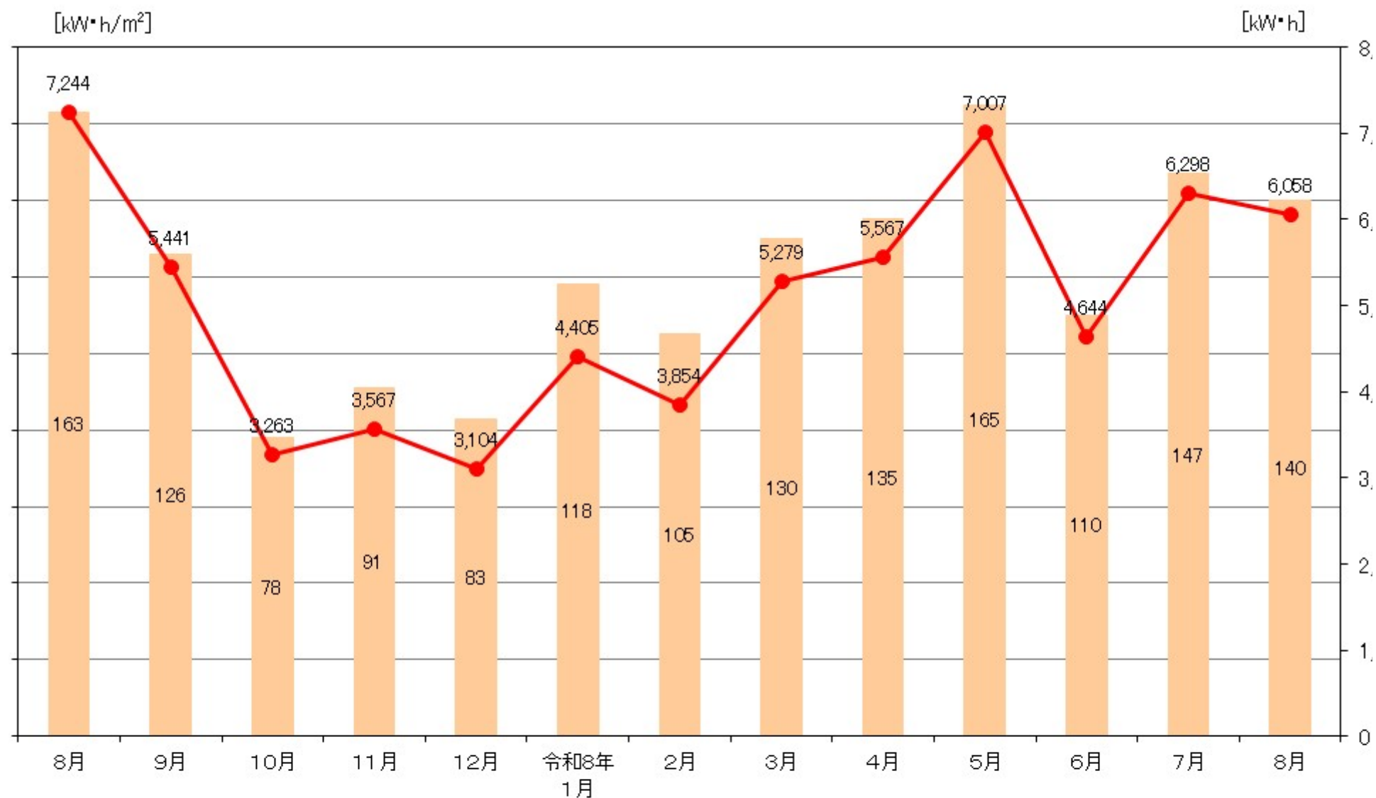
図. 市役所にある太陽光発電システム(60kW)の発電量と日射量との関係 (令和7年8月～令和8年8月)
