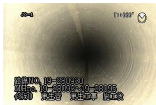
更生工事後の内面
