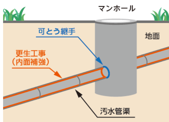
耐震化部分図
