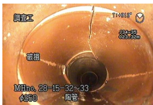
更生工事前の内面
